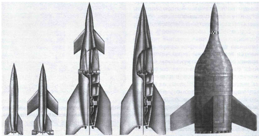
Проекты баллистических ракет А-4, крылатой А-4b, МБР А-9/А-10, А-11 и трехступенчатой А-12 конструкции Вернера фон Брауна. 1937-1944 гг.
