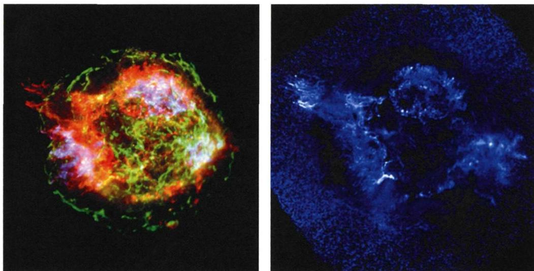
Остаток вспышки сверхновой Cas A (слева). Внешние зеленые области в форме кольца являются следствием воздействия прямой ударной волны. Внутри этого кольца выброшенное вещество нагрето до 10^6 K обратной ударной волной (Хванг и др., 2004). Изображение получено с помощью обсерватории "Чандра" в разных диапазонах энергий: красный - в линии кремния Si XIII He \alpha (1,78-2,0 кэВ), зеленый - излучение в континууме 4,2-6,4 кэВ. Справа: отношение изображений, полученных в линии кремния и континууме в диапазоне энергий 1,3-1,5 кэВ, демонстрирующее выброс и контрвыброс. Последние хорошо прослеживаются по излучению кремния. (NASA/CXC/GSFC/U Hwang et al.).
