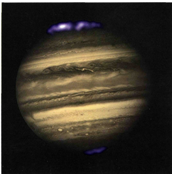
Комбинированное изображение Юпитера, полученное космическим телескопом им. Хаббла и обсерваторией "Чандра". Хорошо видно мощное авроральное рентгеновское излучение из околополярных областей. (X-ray: NASA/CXC/SwRI/R. Gladstone et al.; Optical: NASA/ESA/Hubble Heritage, AURA/STScI).
