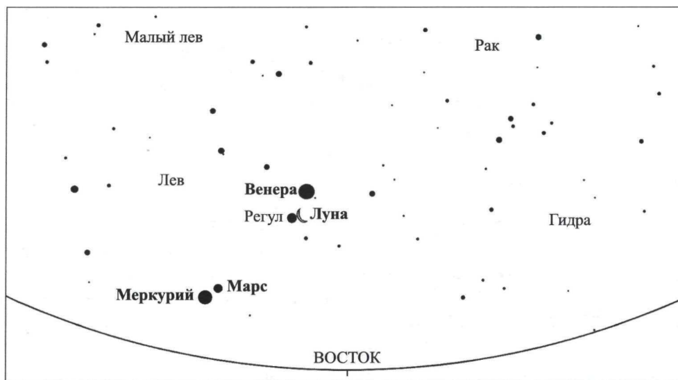
Вид восточной части звездного неба в Москве 18 сентября 2017 г. в 05 ч 00 м по московскому времени. Отмечены положения Меркурия, Марса, Венеры, звезды Регул (α Льва) и Луны.
