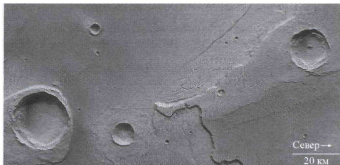
Система каналов Долины Касэй (Kasei Valles) на Равнине Хриса (Chryse Planitia) со следами древнего крупного наводнения. Справа вверху расположен 25-км кратер Вустер (Worcester Crater) с "островом" из вулканического вещества в центре. В середине видны каналы и обрывы, образованные потоками талой воды. Снимок получен 4 марта 2017 г. с помощью АМС "Марс Экспресс". Фото NASA/JPL.
