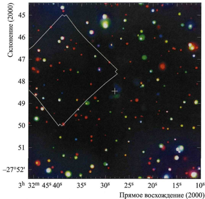
Изображение внутренней части (8'x8') области CDFS, полученное за 4 млн секунд наблюдений обсерватории "Чандра". Разными цветами показаны изображения в разных диапазонах энергий: 0,5-2 кэВ (красный), 2-4 кэВ (зеленый), 4-8 кэВ (синий). Квадратом показана область ультраглубокого поля наблюдений космического телескопа им. Хаббла. (Из работы Ксуе и др., 2011).
