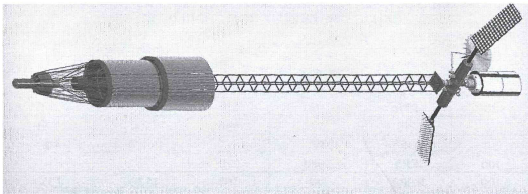
Межорбитальный электроракетный буксир "Геркулес" с термоэмиссионной ядерно-энергетической установкой электрической мощностью 500-600 кВт.
