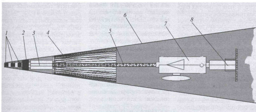
Схема межпланетного транспортного корабля с ядерным электроракетным двигателем: 1 - реакторы ядерной энергетической установки (термоэмиссионные реакторы-преобразователи), 2-тенивая радиационная защита, 3-отсек оборудования ЯЭУ, 4-холодильник-излучатель, 5-трансформируемая ферма, 6-граница конуса радиационной тени, 7-полезный груз, 8-электроракетная двигательная установка (высоковольтная).
