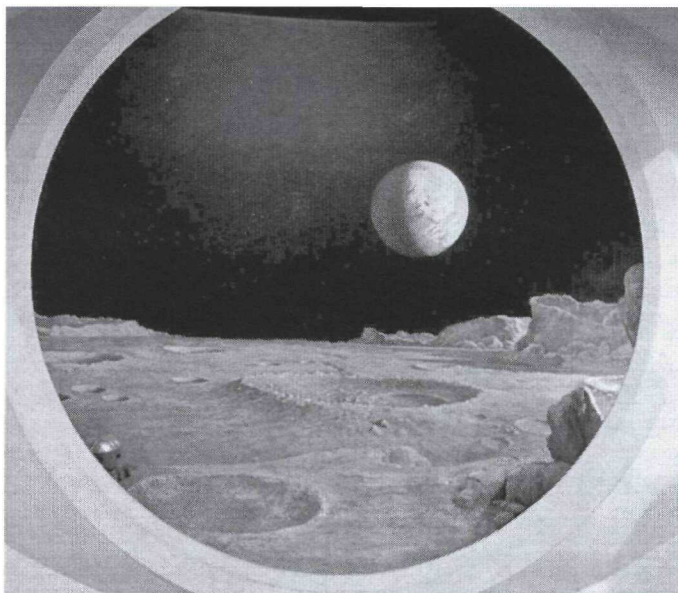
Диорама Луны.
