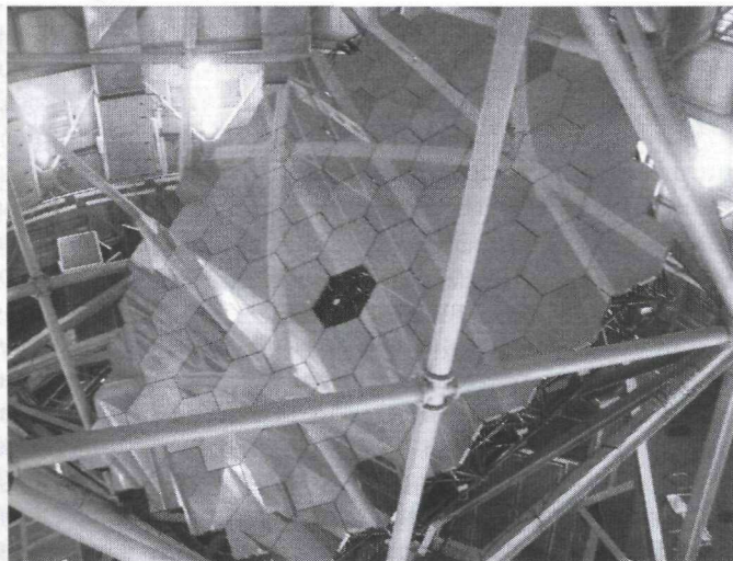
Составное зеркало телескопа SALT. Виден отсутствующий сегмент, который снят для обновления зеркального покрытия.
