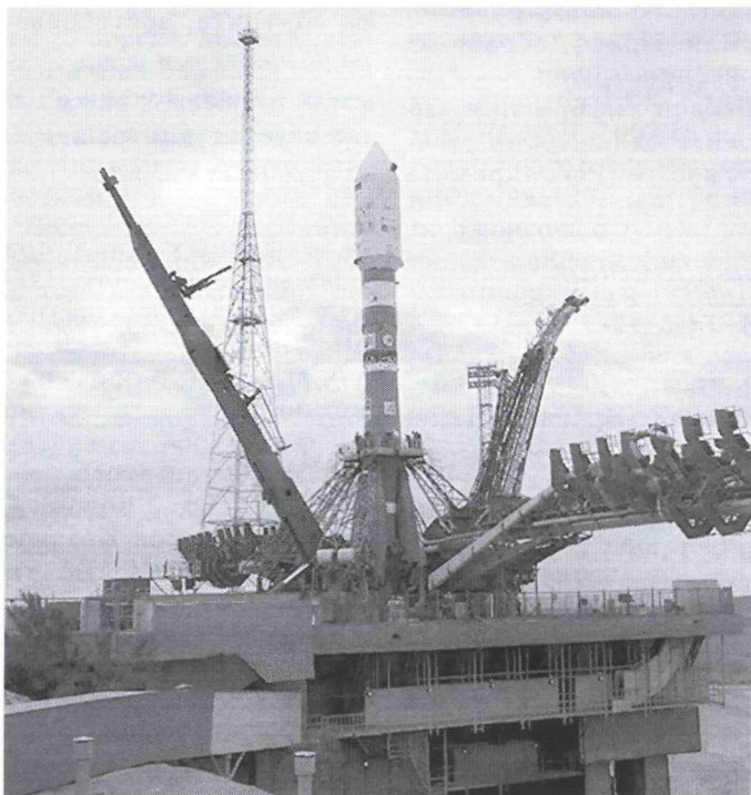
Ракета-носитель "Союз-2.1а" с космическим аппаратом дистанционного зондирования Земли "Канопус-В-ИК". Космодром Байконур, июль 2017 г. Фото Госкорпорации "Роскосмос".
