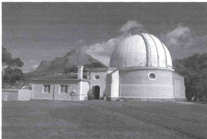
Здание телескопа Мак-Клейна. На заднем плане видна угловая часть Столовой горы -Пик Дьявола
