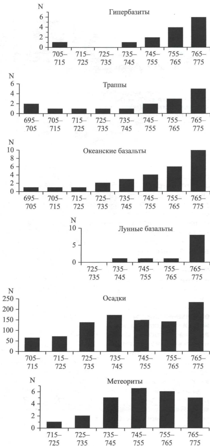
Графики данных терромагнитного анализа. Гистограммы точек Кюри (в градусах Цельсия) демонстрируют однообразие составов металлического железа земного и внеземного происхождения. N - число образцов в данном температурном интервале.
