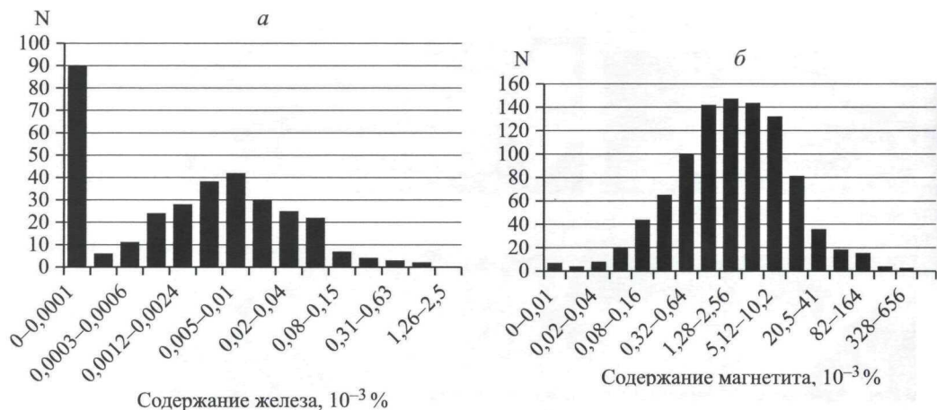
Графики концентрации частиц металлического железа и магнетита в осадочных породах по данным термомагнитного анализа. N-число определений.
