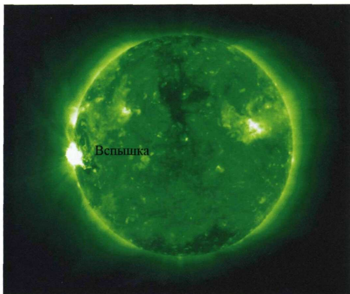
Вспышка (возможно, большая) 23 июля 2017 г. на невидимой с Земли стороне Солнца, по наблюдениям космической солнечной обсерватории "STEREO-A" в линии крайнего ультрафиолета Fe XII ( \lambda = 195 \text{ \AA} ; http://www.solarmonitor.org/ ).
