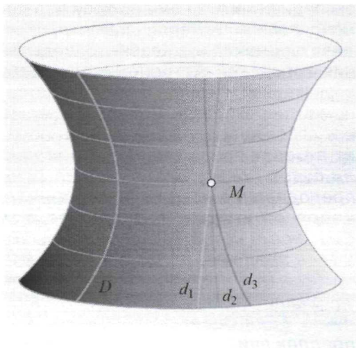
Параллельные прямые пересекаются в искривленном пространстве.
