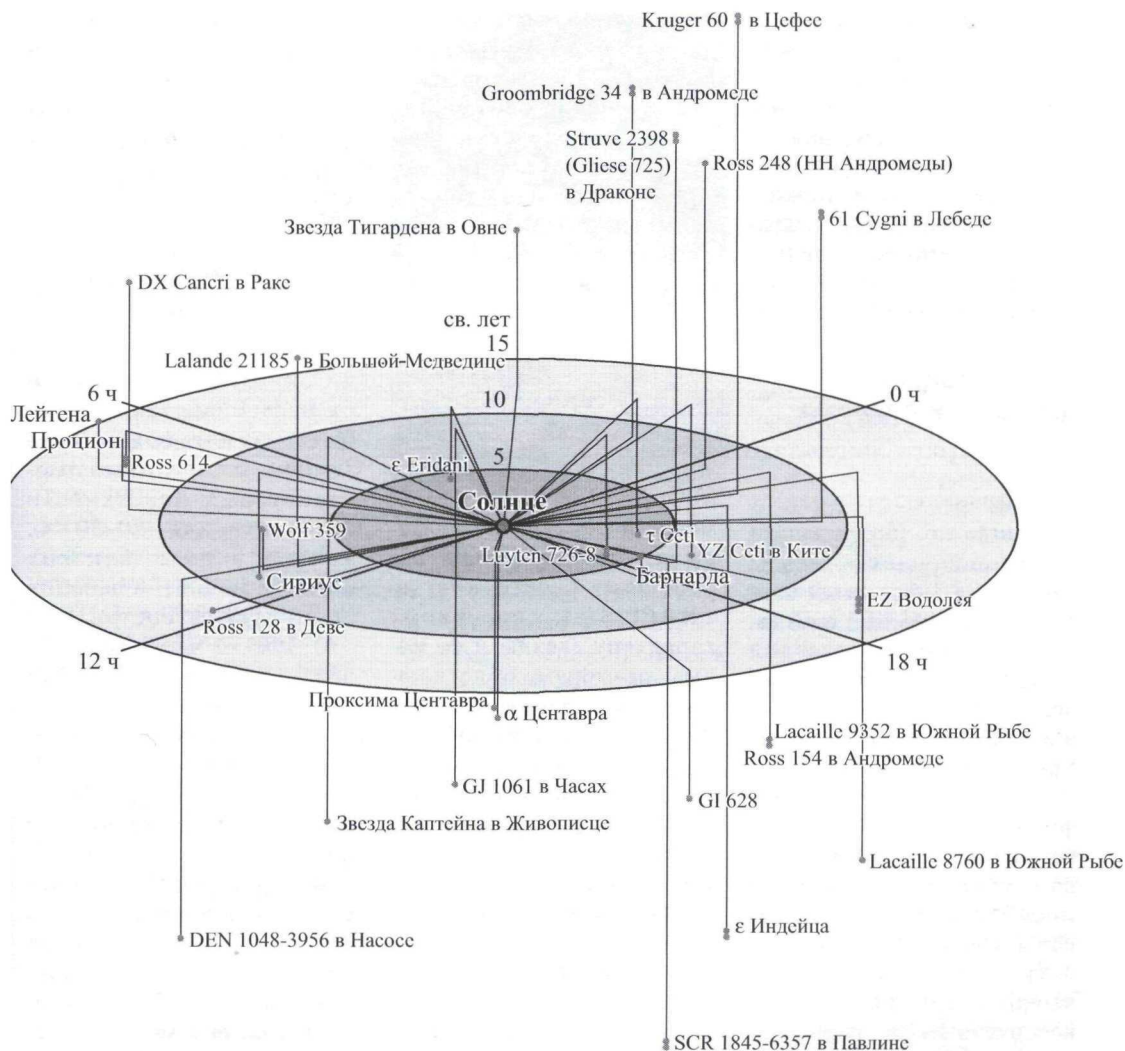
Расположение ближайших к Земле звезд (схема). В пределах 14 св. лет от Земли их насчитывается около нескольких десятков. Это число приближается к тысяче с увеличением расстояния от нашей планеты (до 40 св. лет).
