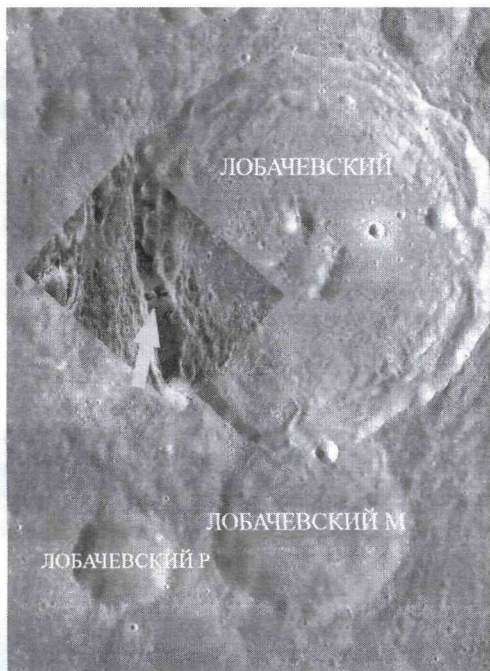
Комплекс кратера Лобачевский на обратной стороне Луны. На внешнем краю кратера были обнаружены структуры (обозначены стрелкой), похожие на очертания башен или столбов. Фото NASA.
