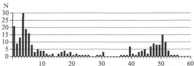
Графики данных микрозондового анализа. Диаграмма концентрации никеля (%) в металлической части каменных метеоритов. N-число измерений. Большое расхождение процентного содержания никеля от измерения к измерению - результат, главным образом, гравитационной дифференциации вещества планеты.
