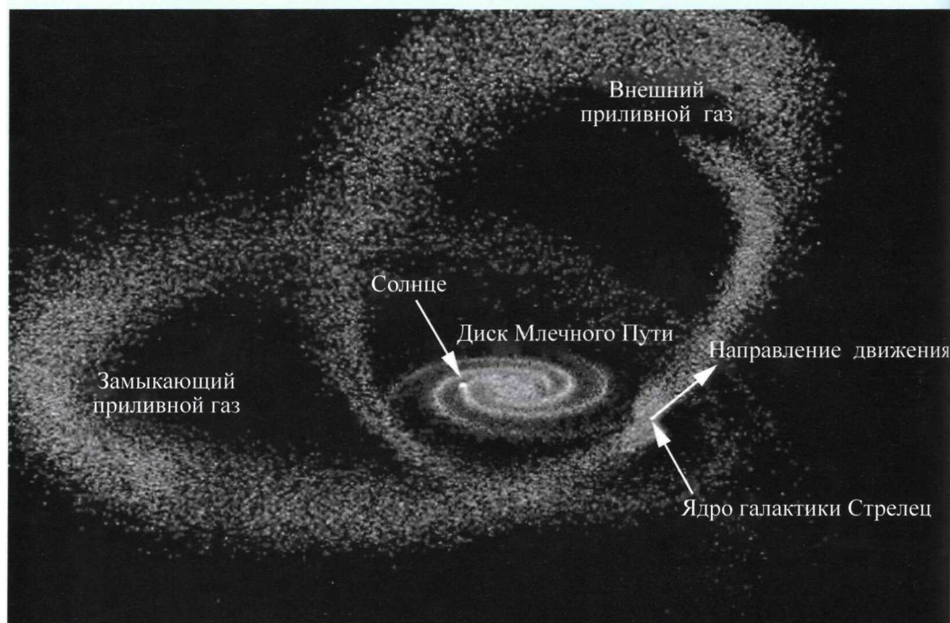
Схема расположения в пространстве Млечного Пути и петлеобразной карликовой галактики Стрелец.
